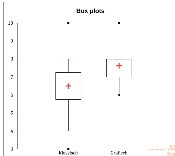
Abbildung 77: Boxplot praktisch
