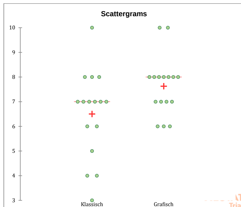
Abbildung 78: Punkteverteilung praktisch
