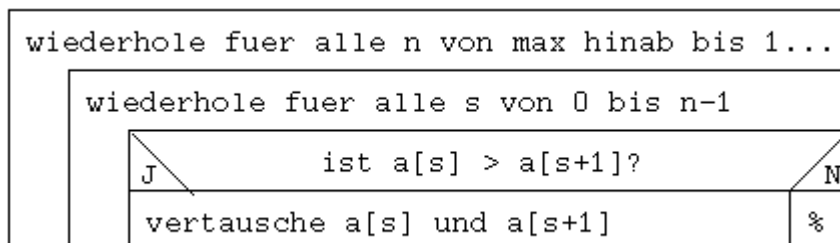
Abbildung 58: Pseudocode [18]
